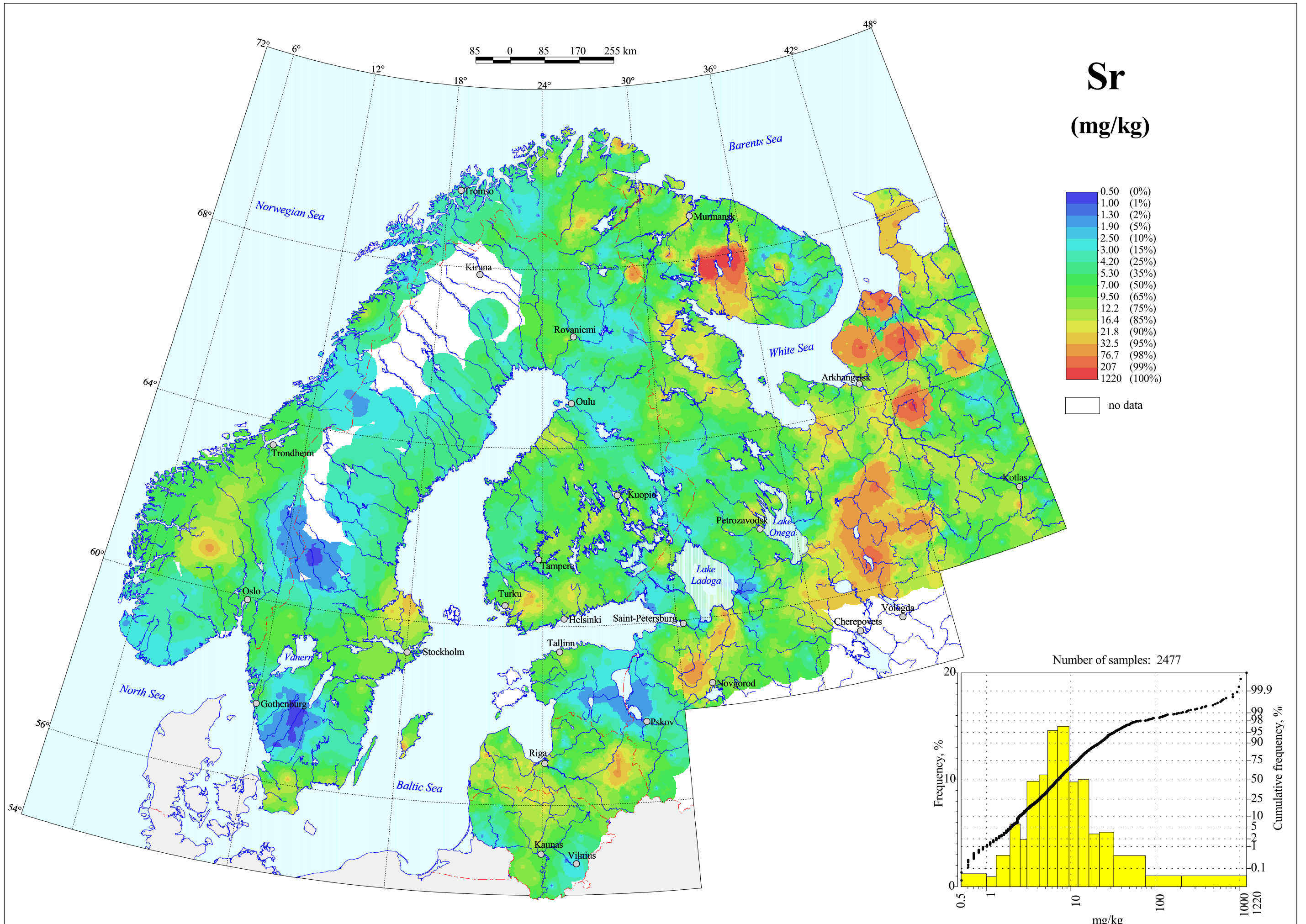
Strontium in C-horizon, Grain Size <2 mm, Aqua regia Extraction
